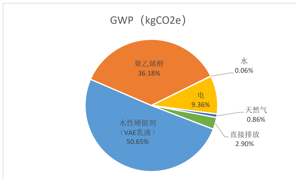
图 4.1 硬挺剂的碳足迹按物质获取展示
