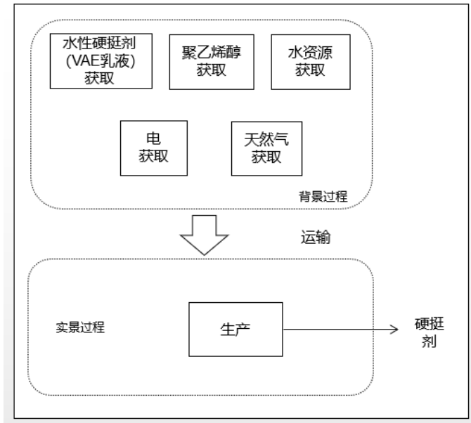
图 1.1 硬挺剂生产系统边界图
