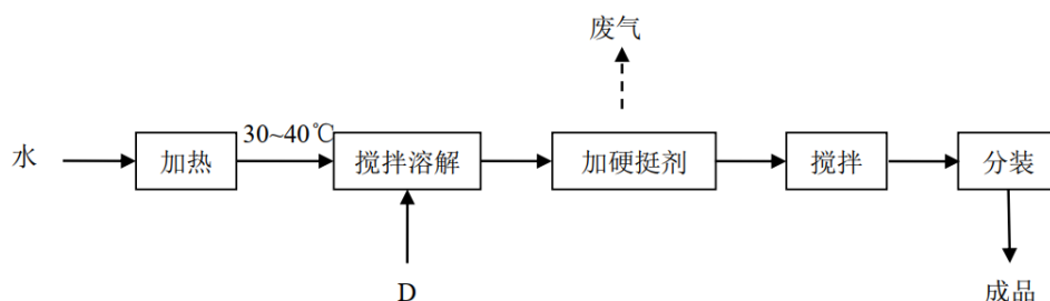
图 3.1 硬挺剂生产工艺流程
